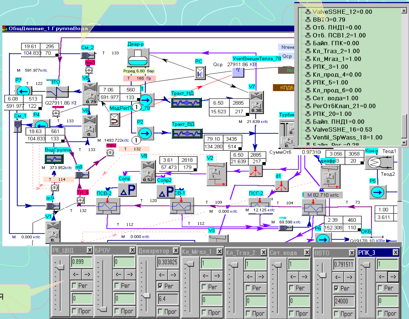
Схема ПГУ 450
