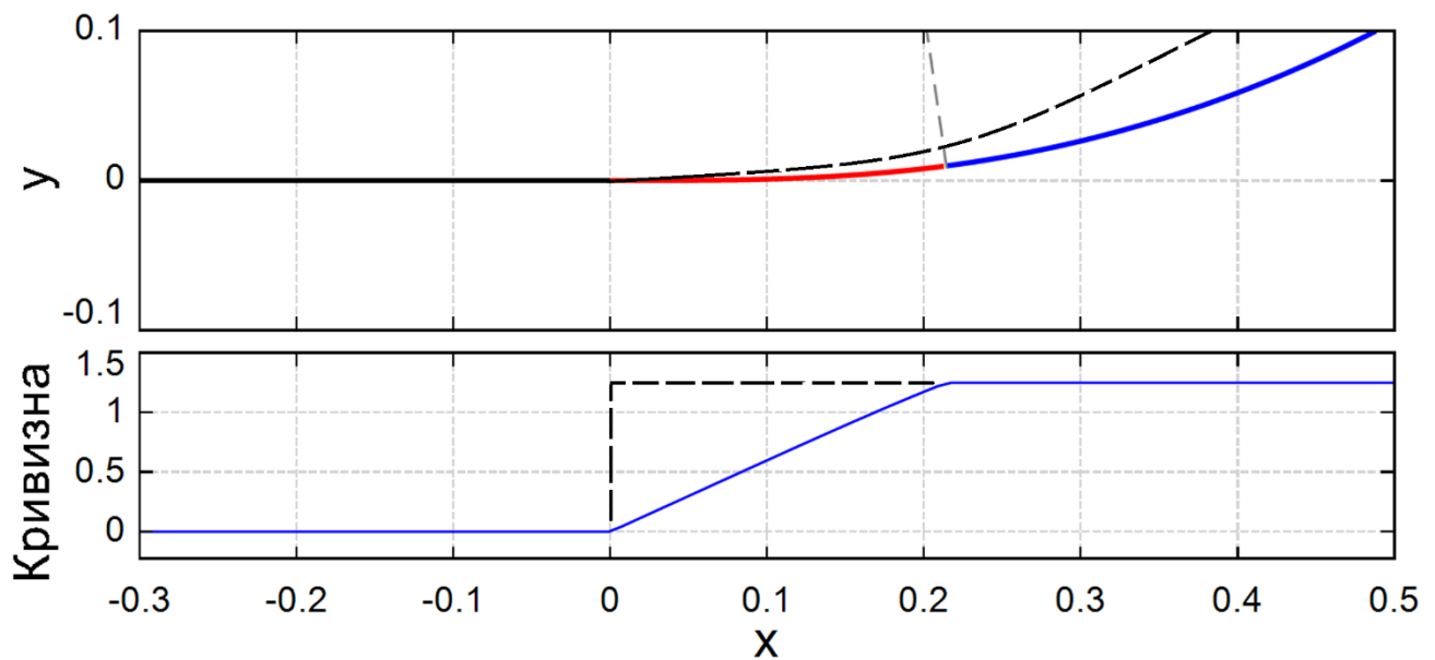
Рис. 1.5. Кривая схода трамвая с прямолинейного на округлый участок (вверху) и её кривизна (внизу); пунктир – это поворот без переходной кривой
