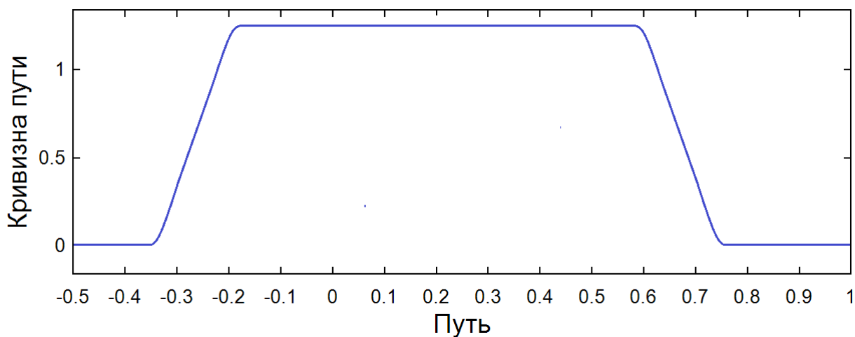
Рис. 1.26. Сглаженная кривизна пути при повороте трамвая
