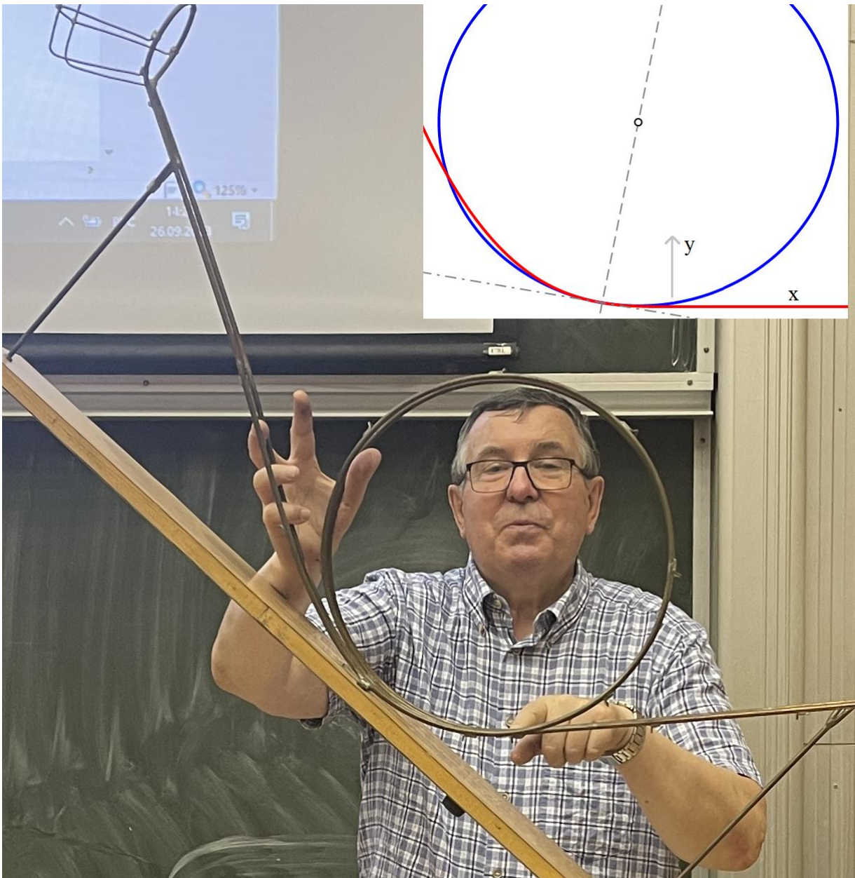
Рис. 1.24. Физическая модель чертовой петли американских горок – лектор показывает на точку, где прямая переходит в кубическую параболу; левее точка, где кубическая параболa переходит в окружность
