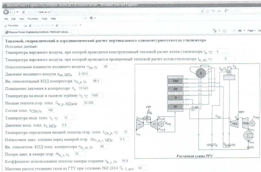
Рис. 2. Фрагмент подготовленного по технологии Mathcad Calculation Server блока исходных данных для расчета котла-утилизатора
