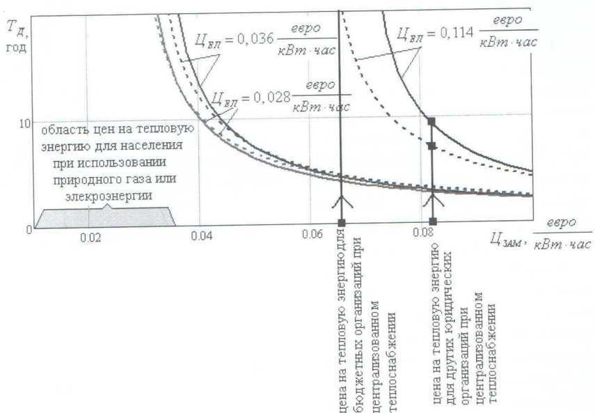
Рис. 5. Влияние цен на дисконтированный срок окупаемости ( T_d ) внедрения теплового насоса в условиях Украины (г. Ровно): тепловый насос покрывает 50% установленной тепловой мощности; сплошные линии – в качестве пикового источника теплоты используется электрический котел; штриховые линии – в качестве пикового источника теплоты используется газовый котел
