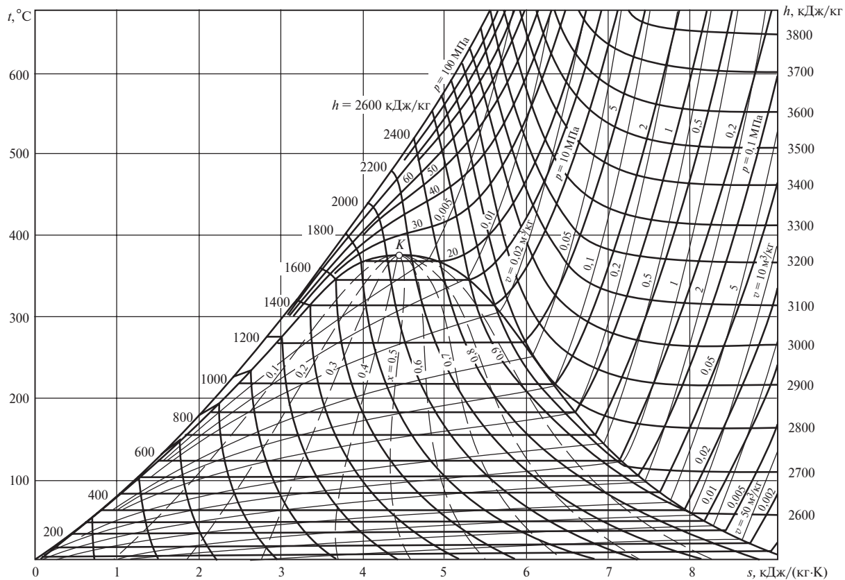
Рис. III. t , s -диаграмма для воды и водяного пара [9]
